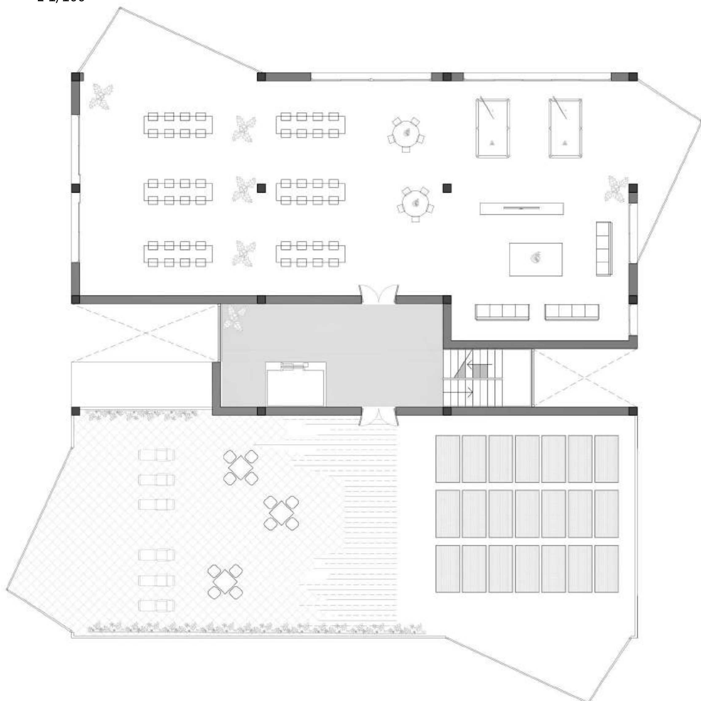
PLANTA COBERTA E 1/100
