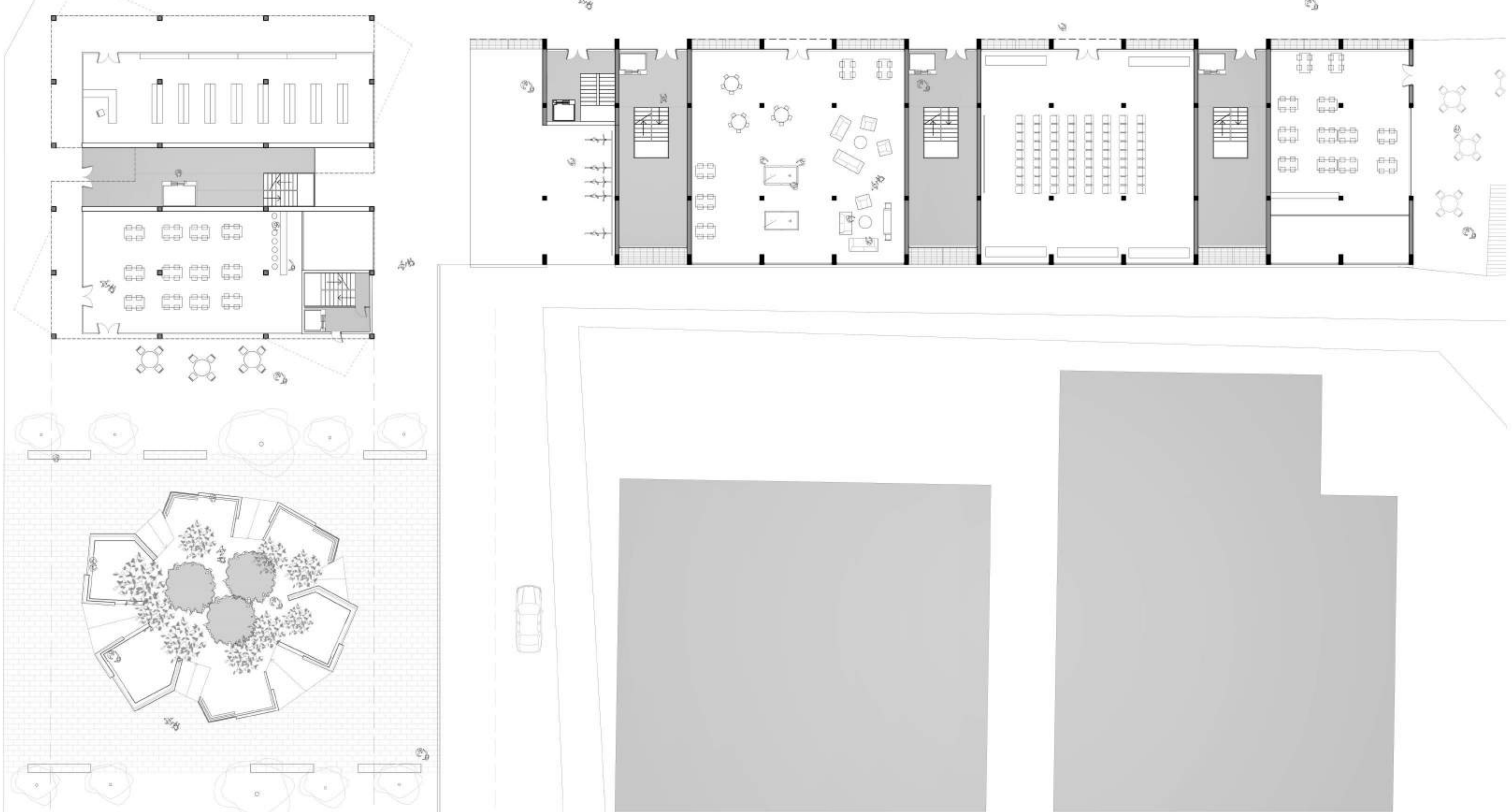
Planta Baixa E 1/200
