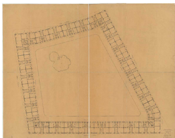
Kay Fisker Edificio de viviendas Gullfosshus, Copenhagen, Dinamarca, 1926-1932
