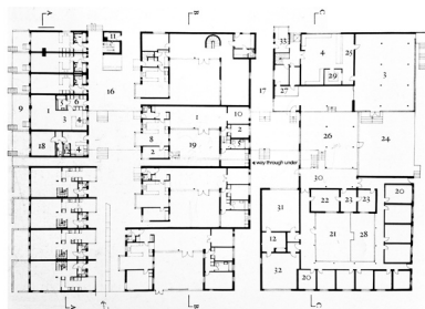
Ralph Erskine Residencia de estudiantes Clare Hall, Cambridge, Reino Unido, 1969-1971
