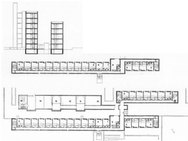
Arne Jacobsen Residencia de estudiantes en Copenhague, Dinamarca, 1969-1970
