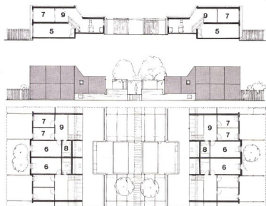
J. P. Storgard, J. Orum-Nielsen, H. Marcussen Conjunto residencial Galgebakken, Dinamarca, 1969-
